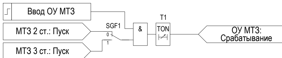
Рисунок 2.24 – Функциональная схема ОУ МТЗ
